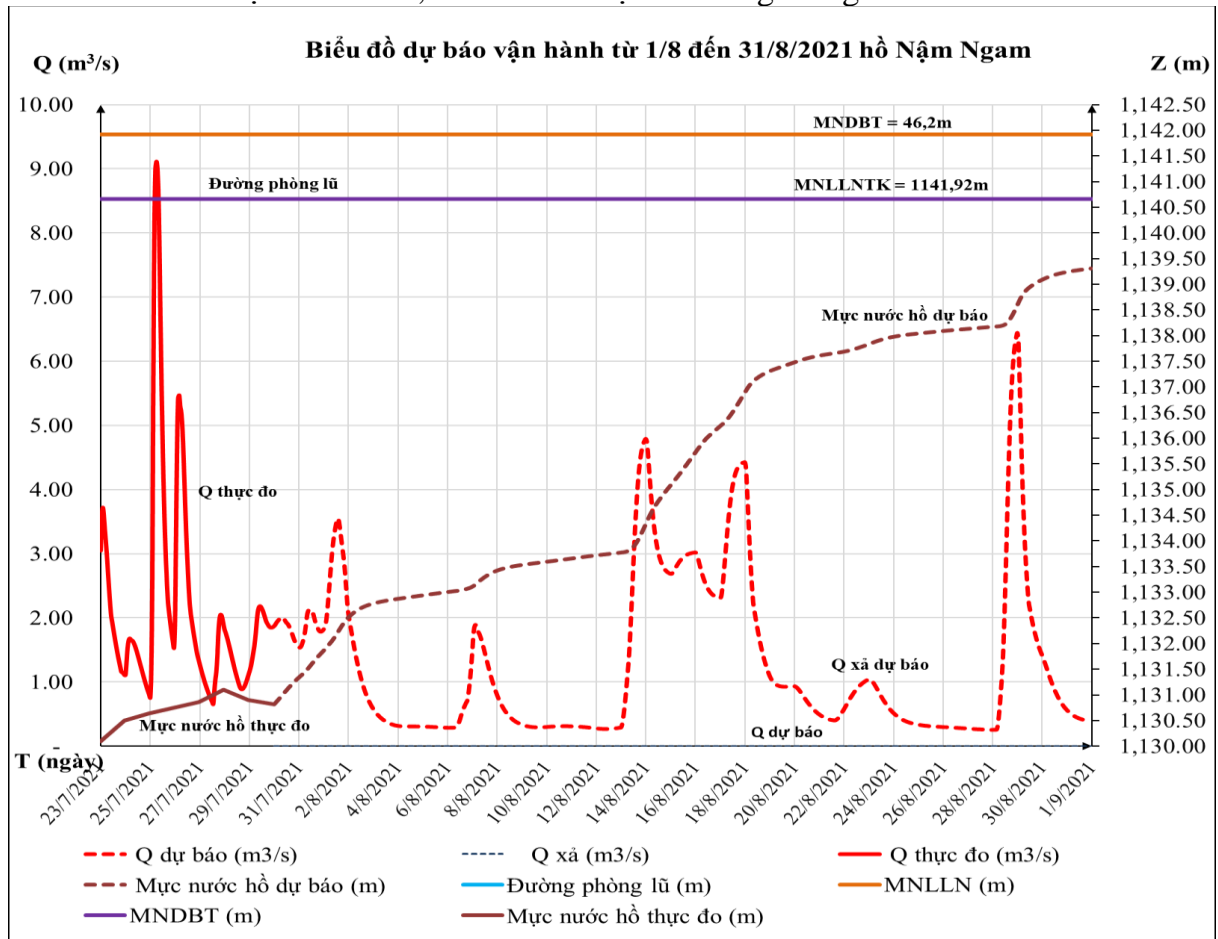
+ Biểu đồ vận hành tích, xả nước hồ dự báo trong tháng 8/2021
